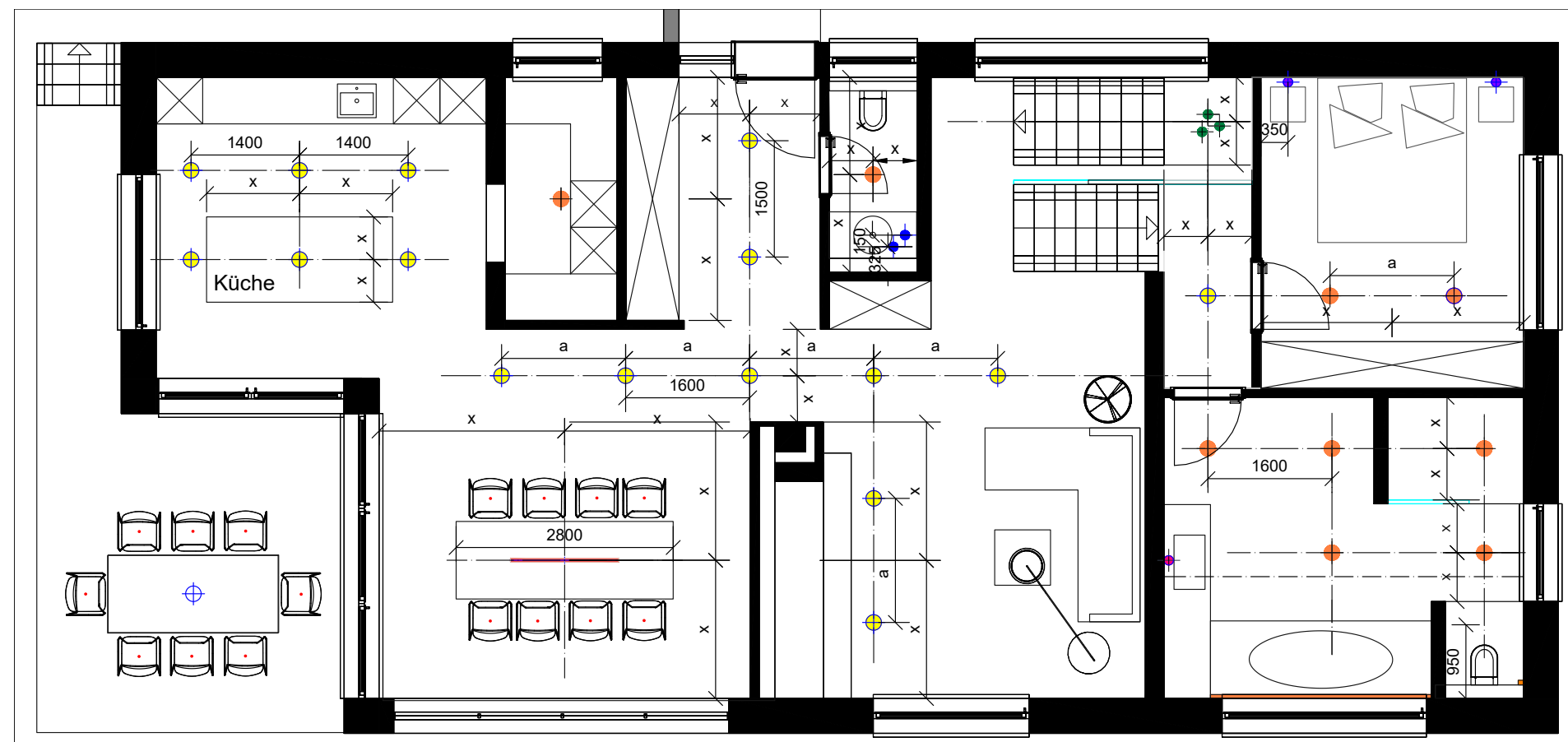
Lichtplanung Grundriss
